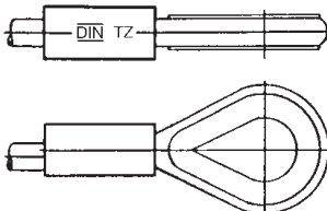
Kennzeichnung (einer Alu-Verpressung)
